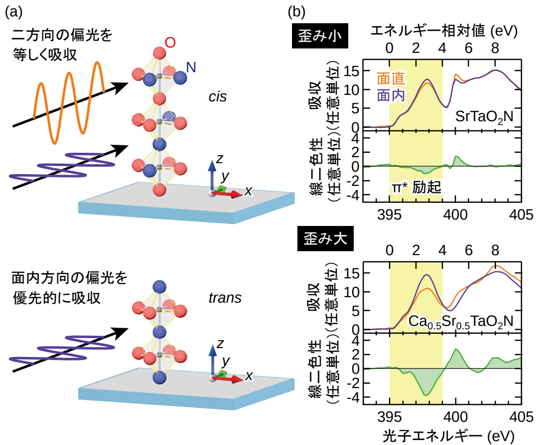
図 3 (a) cis 型構造と trans 型構造の X 線吸収の違い。酸素と窒素の電子軌道の広がる方向はタンタルに対して配位する位置によって変化する。 cis 型の結晶格子がランダムに並んだ状態では縦横両方向に偏光した X 線が等しく吸収されるが、窒素が面直（縦）方向に並んだ trans 型構造では、窒素は面内（横）方向に偏光した X 線をより強く吸収する。(b)歪みの小さな \text{SrTaO}_2\text{N} 薄膜と歪みの大きな \text{Ca}_{0.5}\text{Sr}_{0.5}\text{TaO}_2\text{N} 薄膜で観察された窒素の X 線吸収スペクトル。線二色性は面直偏光の吸収から面内偏光の吸収を引いた差分を表す。
